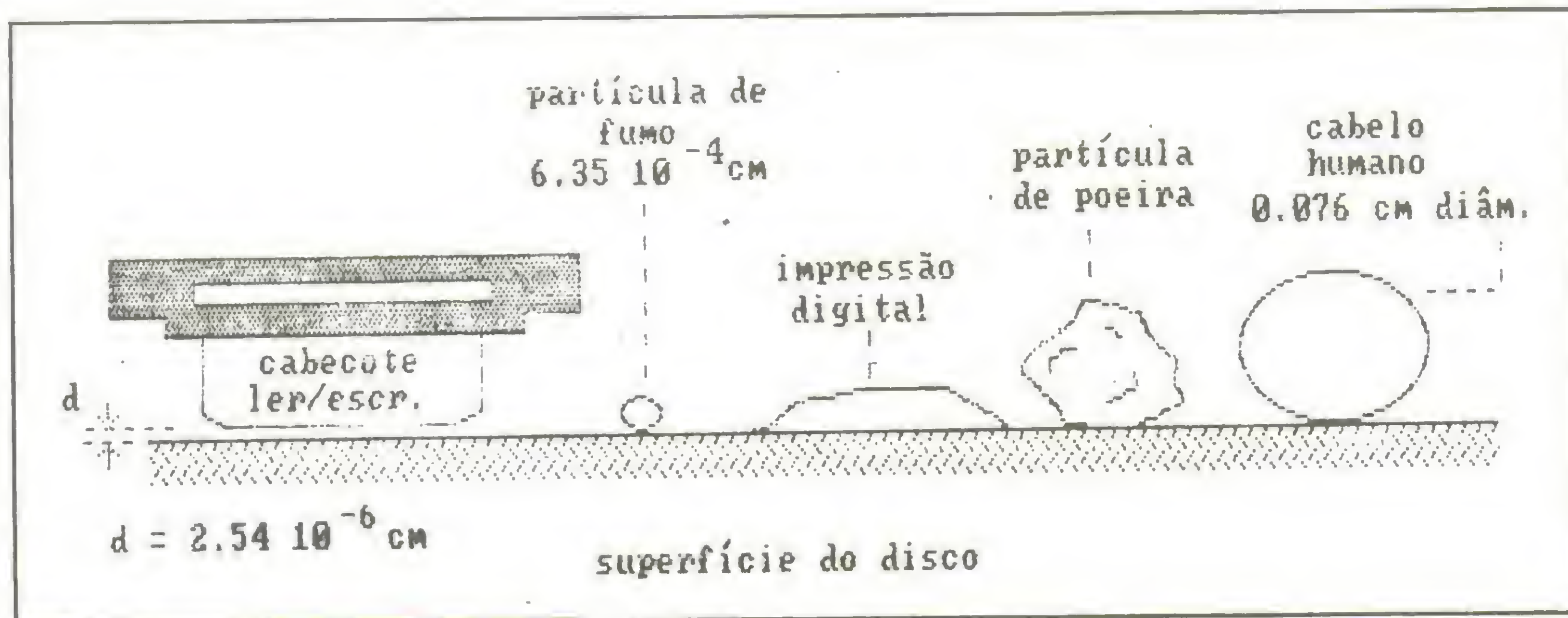
Figura 4 - mostra aproximadamente o afastamento entre a cabeça flutuante do drive e a superfície do disco (cerca de um milionésimo de polegada). Com estas tolerâncias, contaminações tais como partículas de fumo, poeira, impressões digitais ou mesmo o cabelo humano podem tornar o drive inutilizado.
